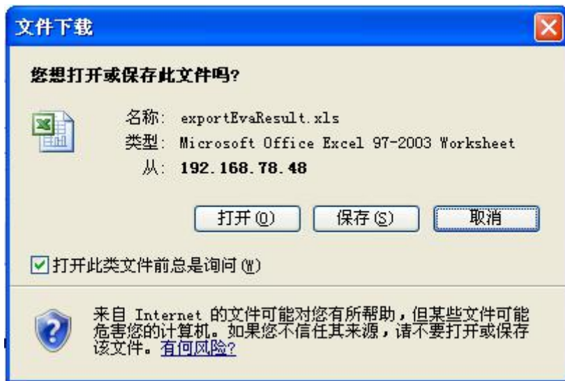
图 5-3-11 对话框
