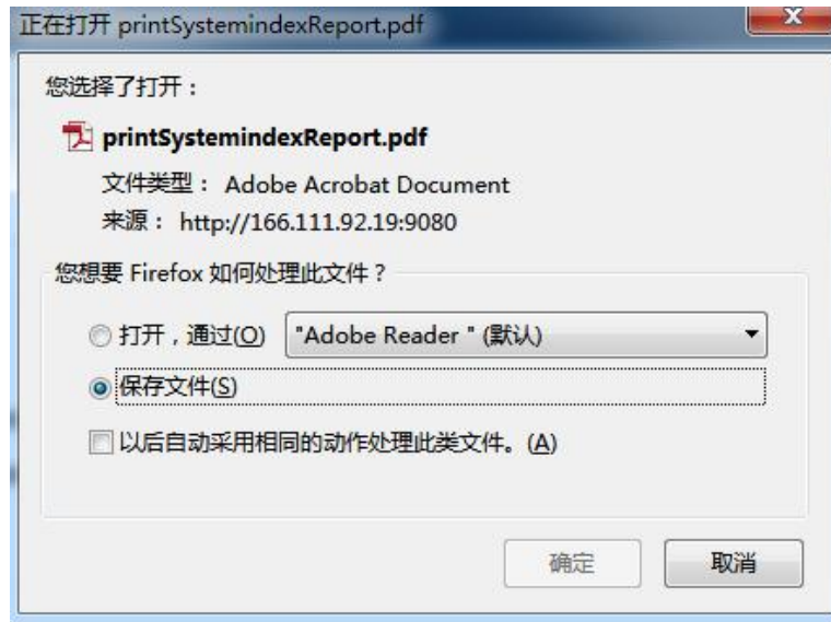
图 4-5-14 对话框
