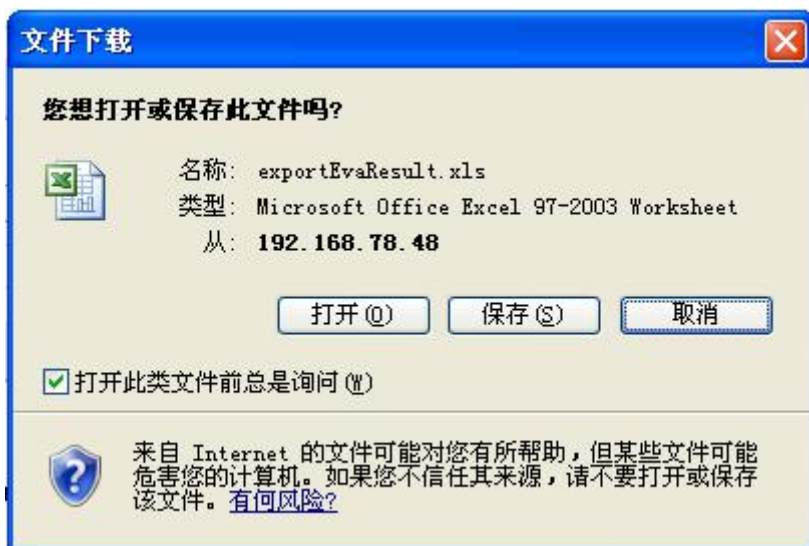
图 4-5-11 对话框
