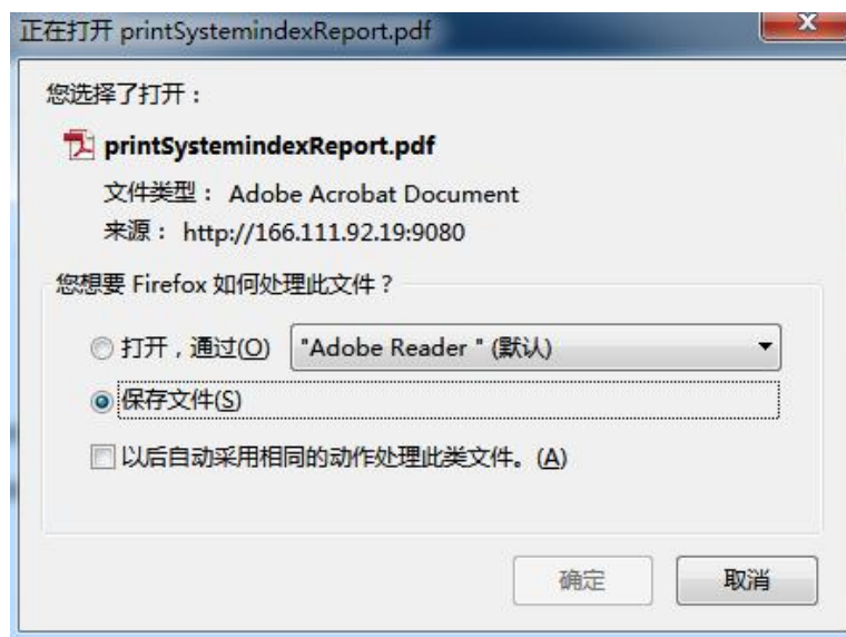
图 4-5-14 对话框
